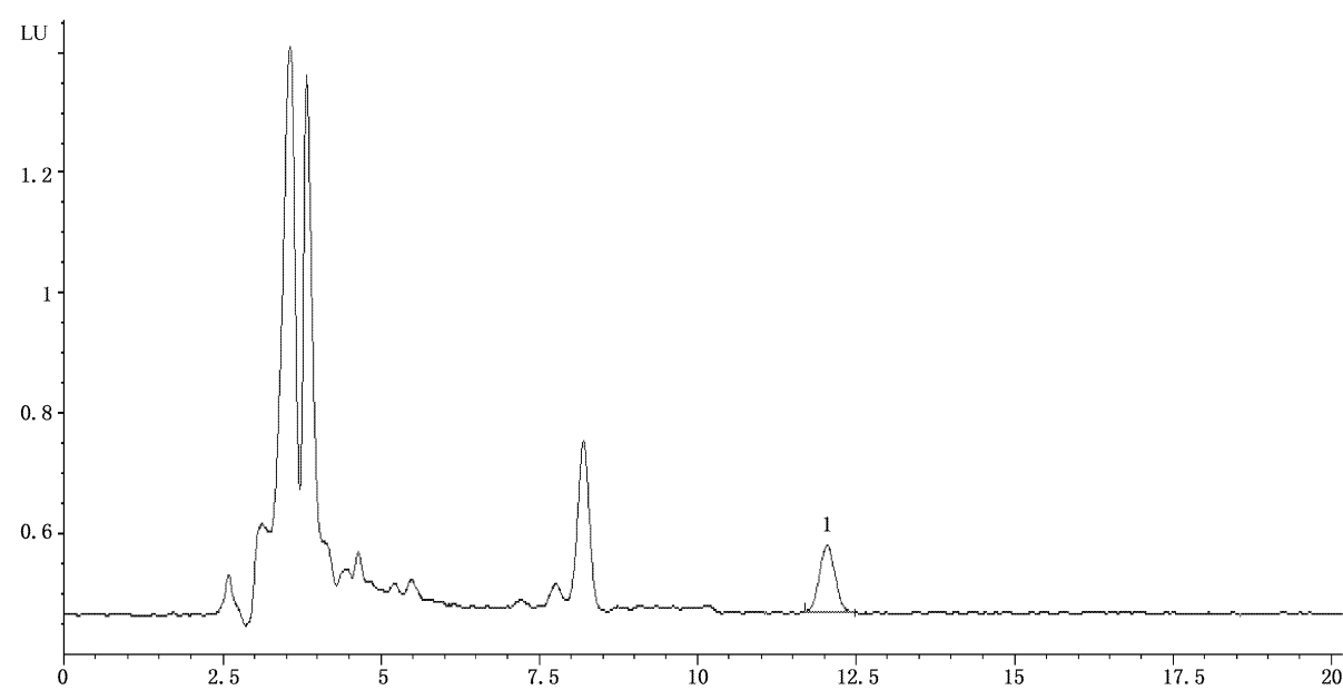
图 A.4 橄榄油中 11-氨基十一酸标准物质衍生物的色谱图
