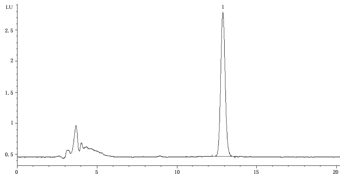
图 A.3 10%(体积分数)乙醇溶液中 11-氨基十一酸标准物质衍生物的色谱图
